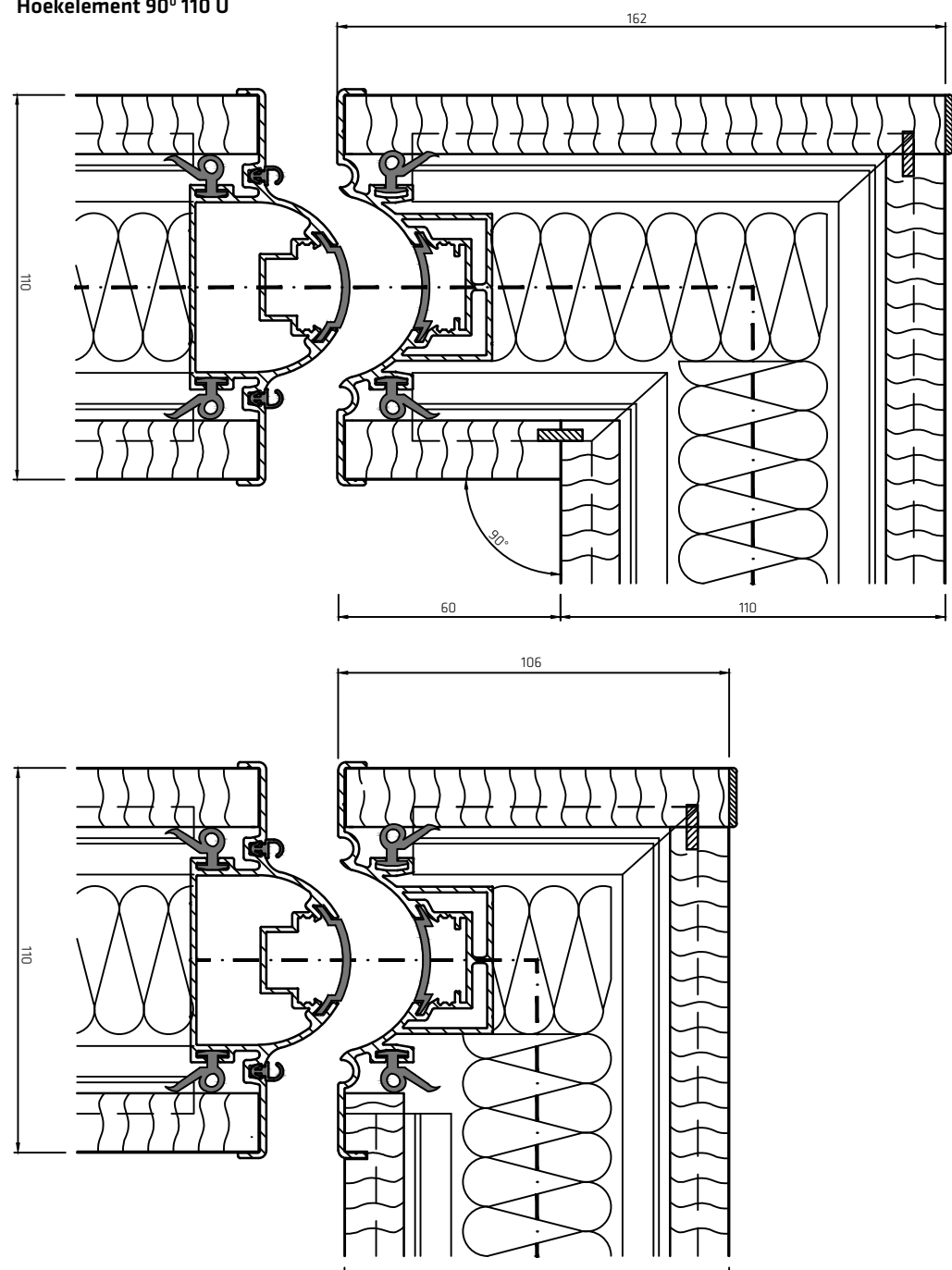
Hoekelament 90° 110 U
