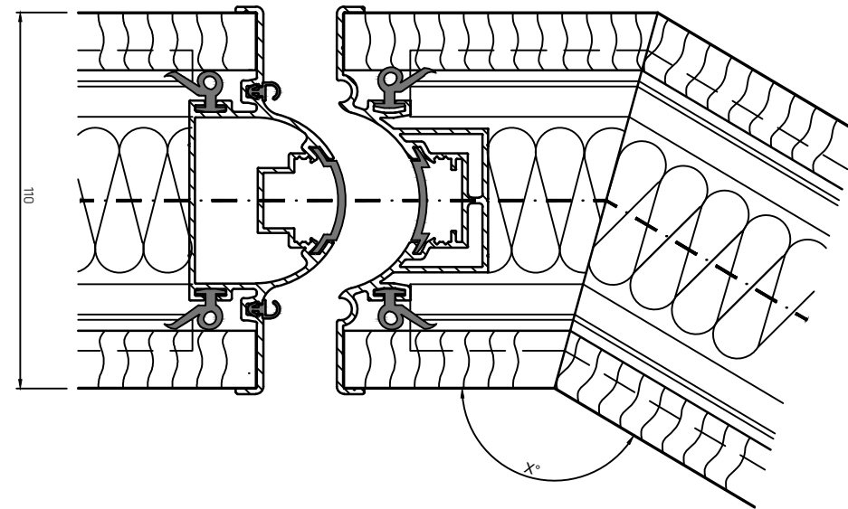
Hoekelement 135° 110 K
