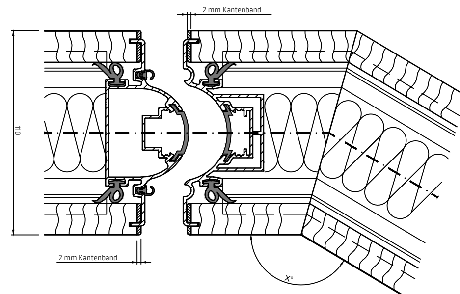
Hoekelement 135° 110 K
