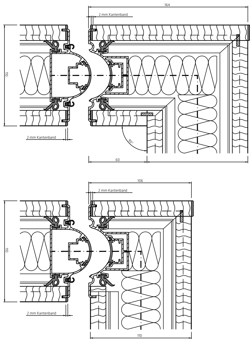
Hoekelament 90° 110 K
