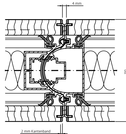
Elementkoppeling 110 K
