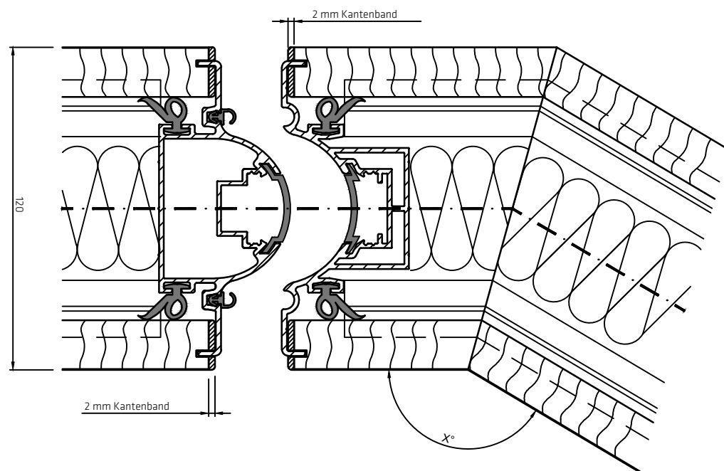
Hoekelement 135° 120 K
