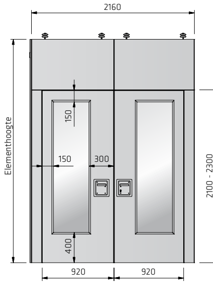
Doorloopdeurelement Voorzien van maximale glasuitsparing
