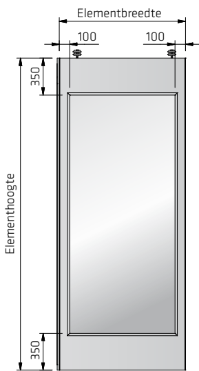
Vensterelement Voorzien van maximale glasuitsparing
