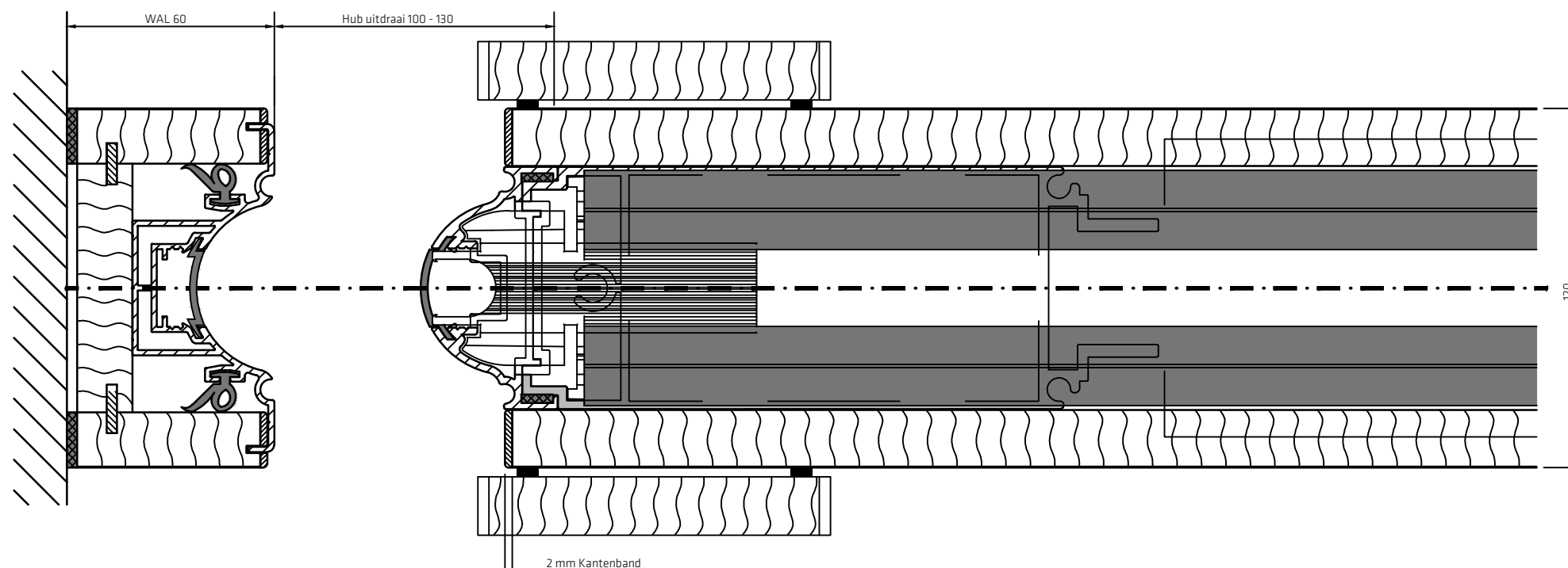
Uitgeschoven met drukbalk
