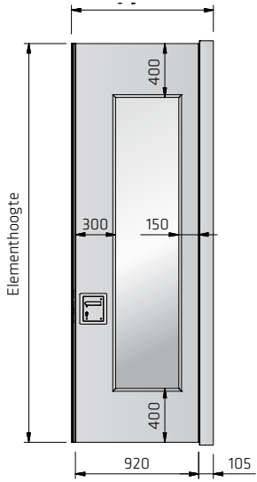
Vastaangeslagen doorloopdeur Voorzien van maximale glasuitsparing
