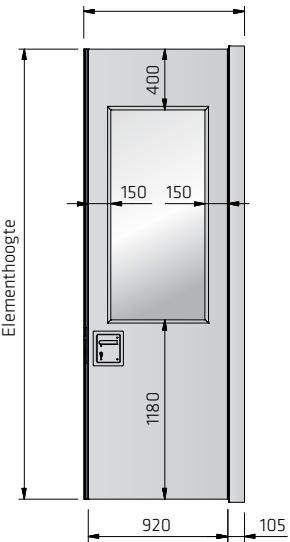
Vastaangeslagen doorloopdeur Voorzien van standaard glasuitsparing
