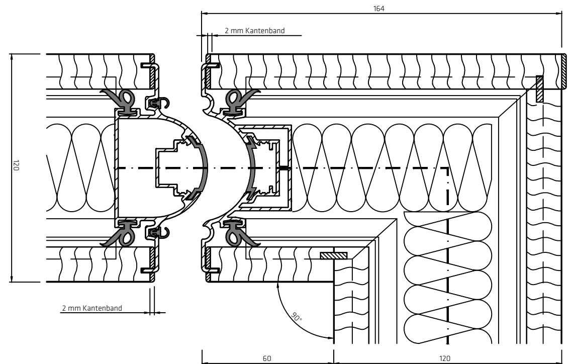
Hoekelement 90° 120 K
