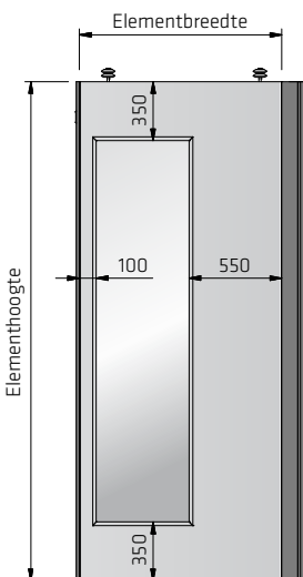
Vensterelement Voorzien van maximale glasuitsparing
