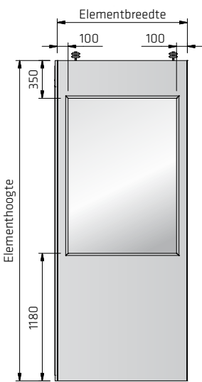
Vensterelement Voorzien van standaard glasuitsparing
