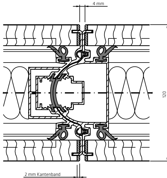
Elementkoppeling 120 K
