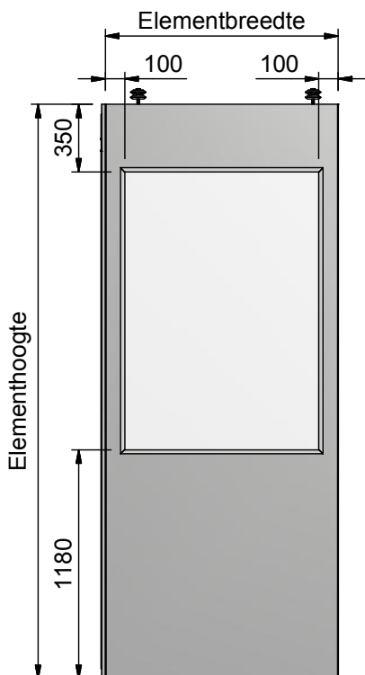
Venster element met standaard glasuitsparing
