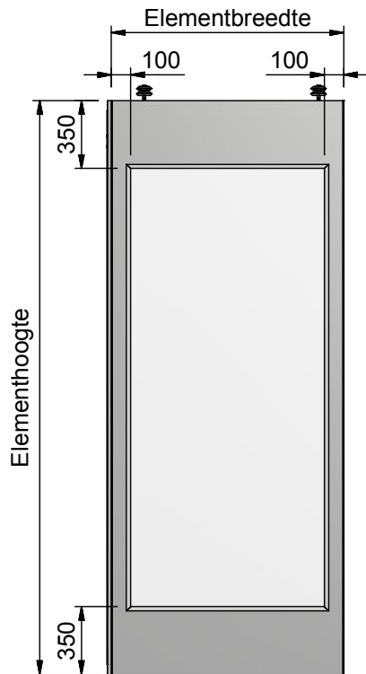
Venster element met maximale glasuitsparing
