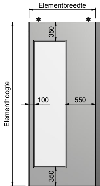
Telescoopelement met maximale glasuitsparing
