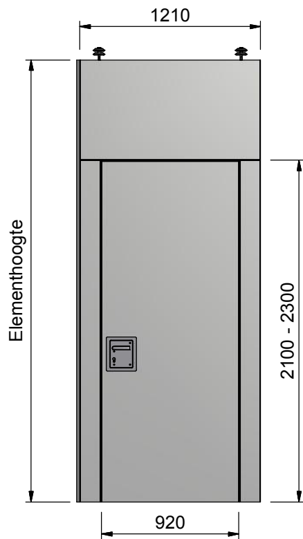
Doorloopdeur element
